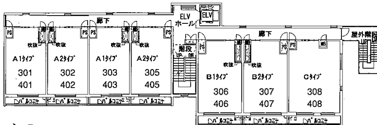
3～4階平面図
