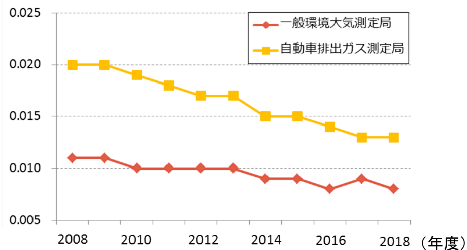
(ppm) 二酸化窒素濃度の年平均値の推移
