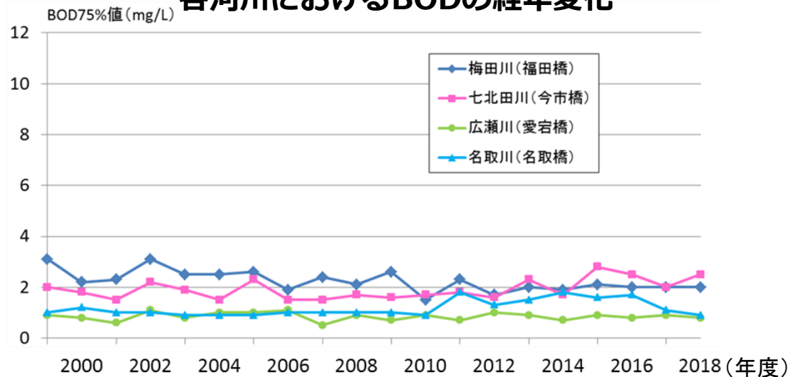
各河川におけるBODの経年変化
