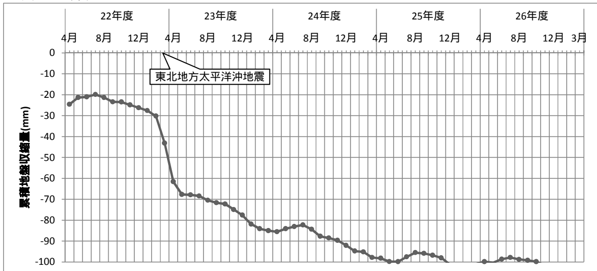
図6.1.3-7(2) 地盤収縮量の変化・日の出町測定局(平成22年4月～平成27年3月)
