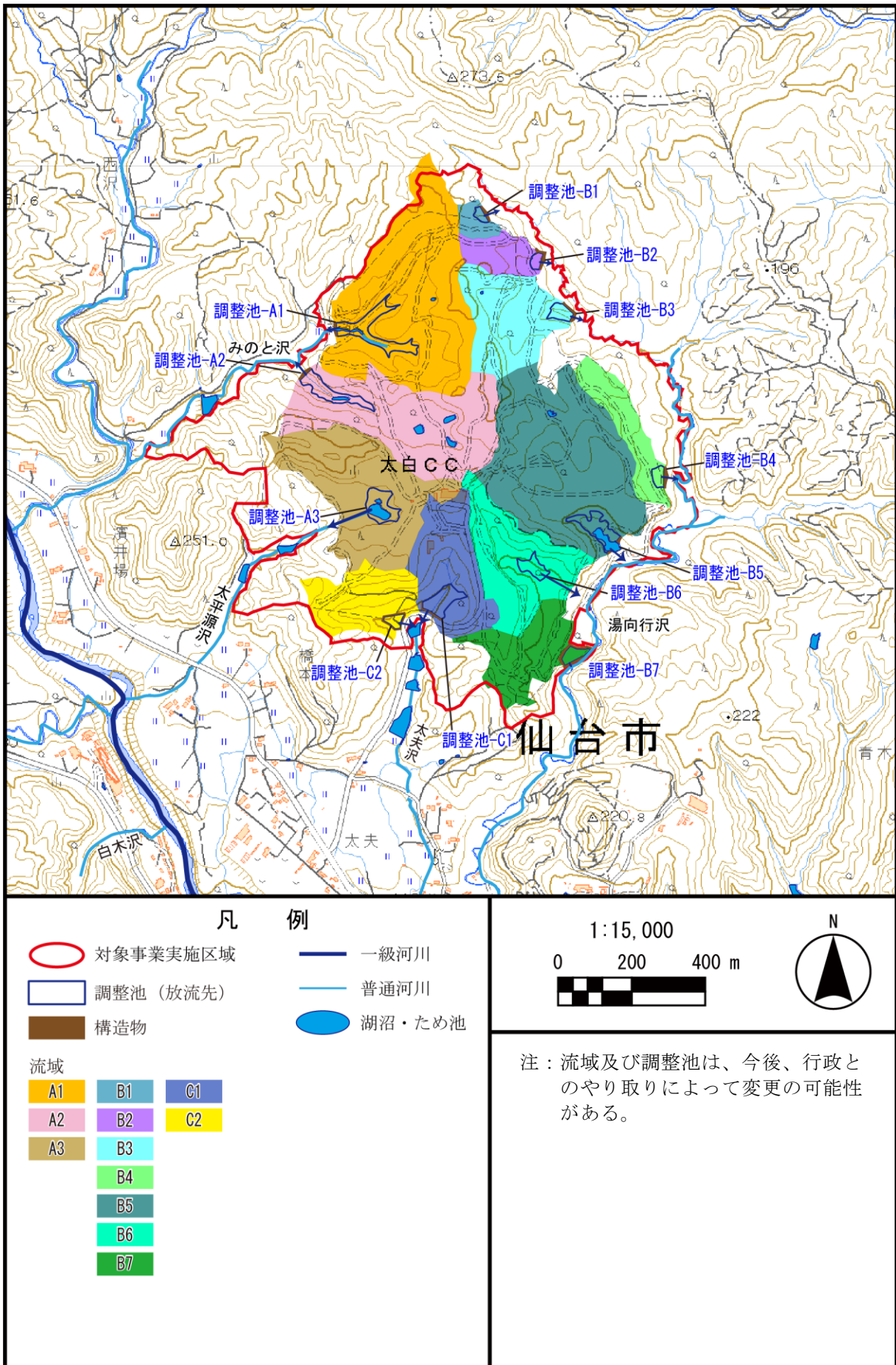
図 2.2-5 調整池の位置、流域及び排水経路
