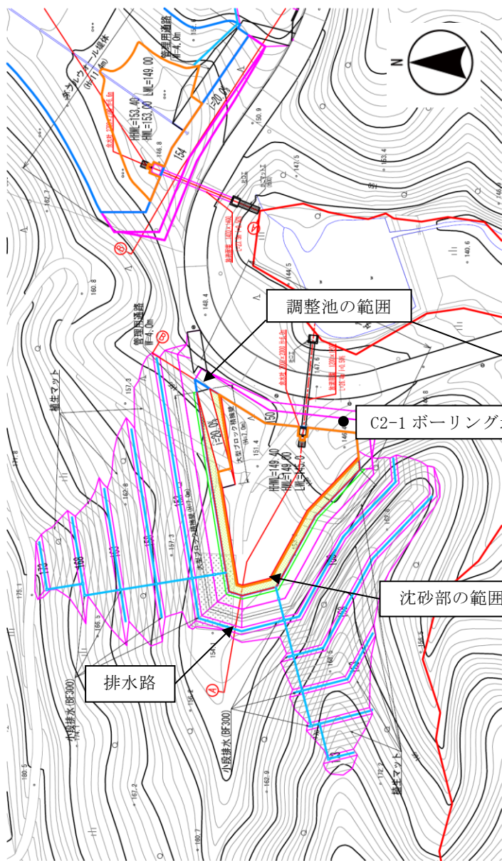
図 2.2-6(12) 調整池の平面図・断面図(C2)
