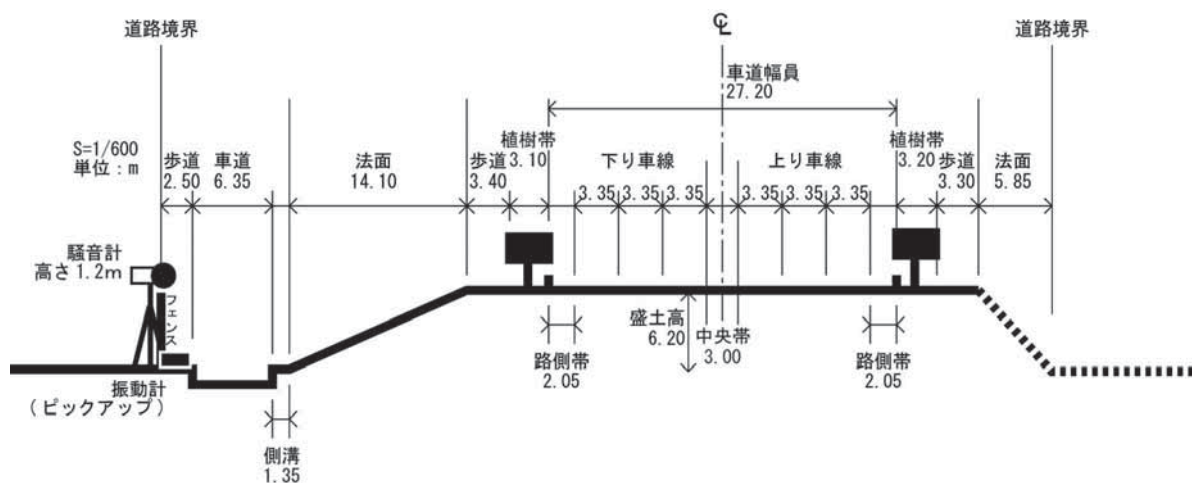
図8.2-2(2) 道路交通騒音調査地点断面図 (No.4~6地点)
