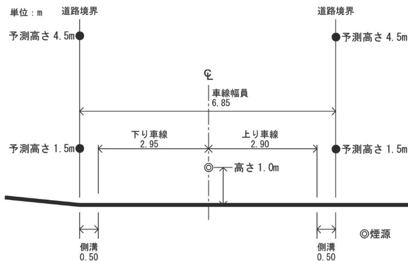
図8.1-23(2) 道路構造と大気質予測地点及び煙源 (No.7~8地点)
