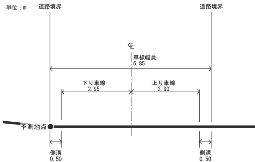
図8.3-5(2) 道路構造及び振動予測地点(No.7~8地点)
