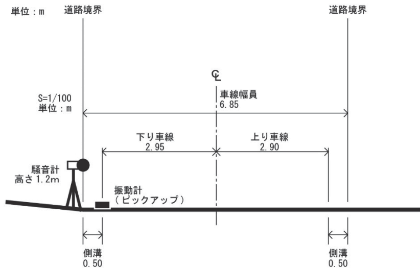
図8.2-2(3) 道路交通騒音調査地点断面図 (No.7~8地点)
