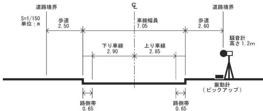
図8.2-2(1) 道路交通騒音調査地点断面図 (No.1～3地点)
