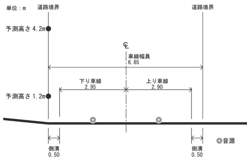
図8.2-11(2) 道路構造と騒音予測地点及び音源位置(No.7~8地点)
