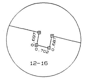
図 I S=1: 100
