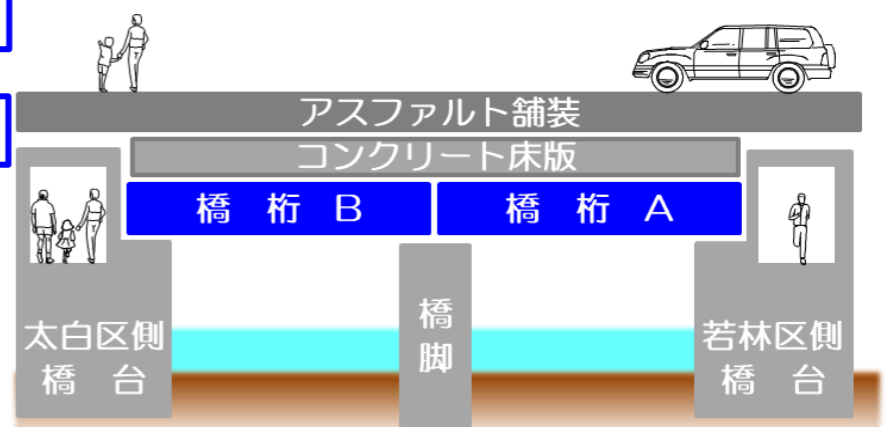
図-1 橋を横から見たイメージ
