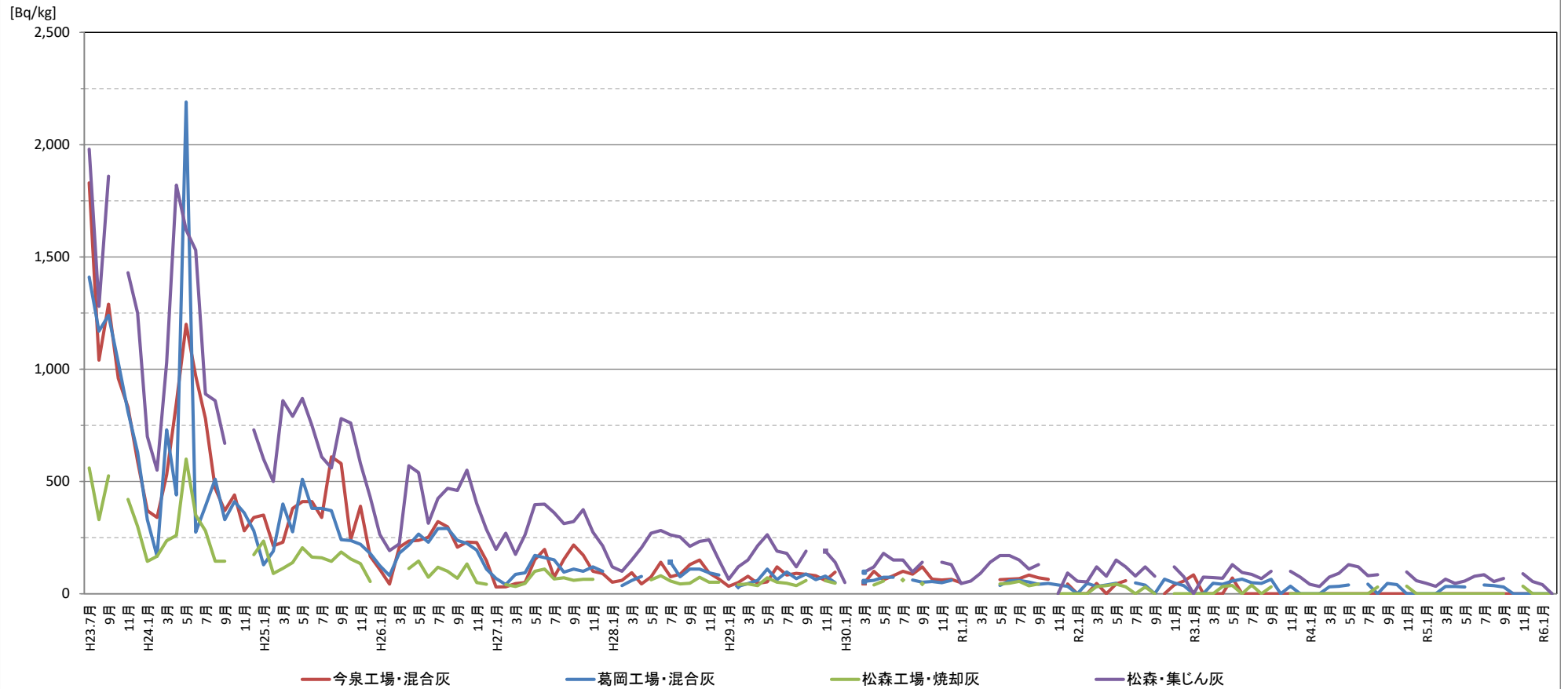
灰の放射性物質濃度の推移 (H23.7~ R6.2)
