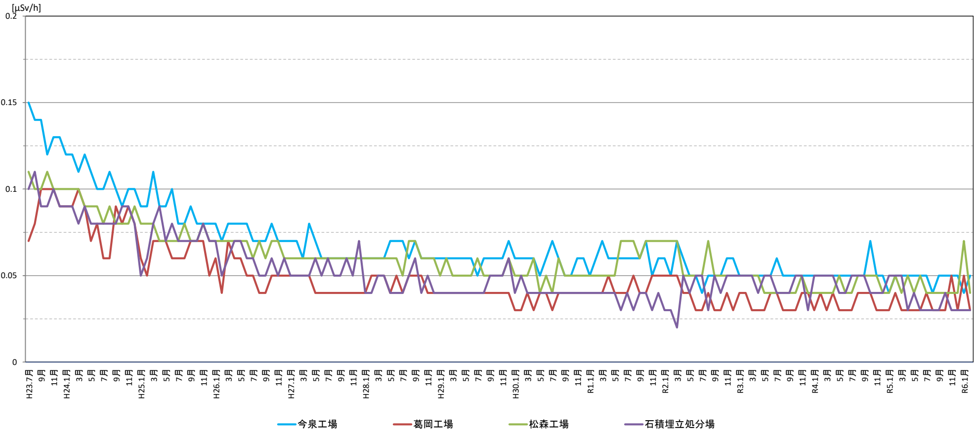
空間放射線量(敷地境界の最大値)の推移 (H23.7~R6.2)
