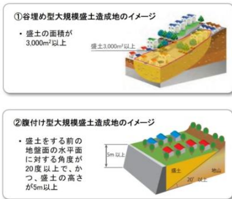
図 8 大規模盛土造成地のイメージ図
