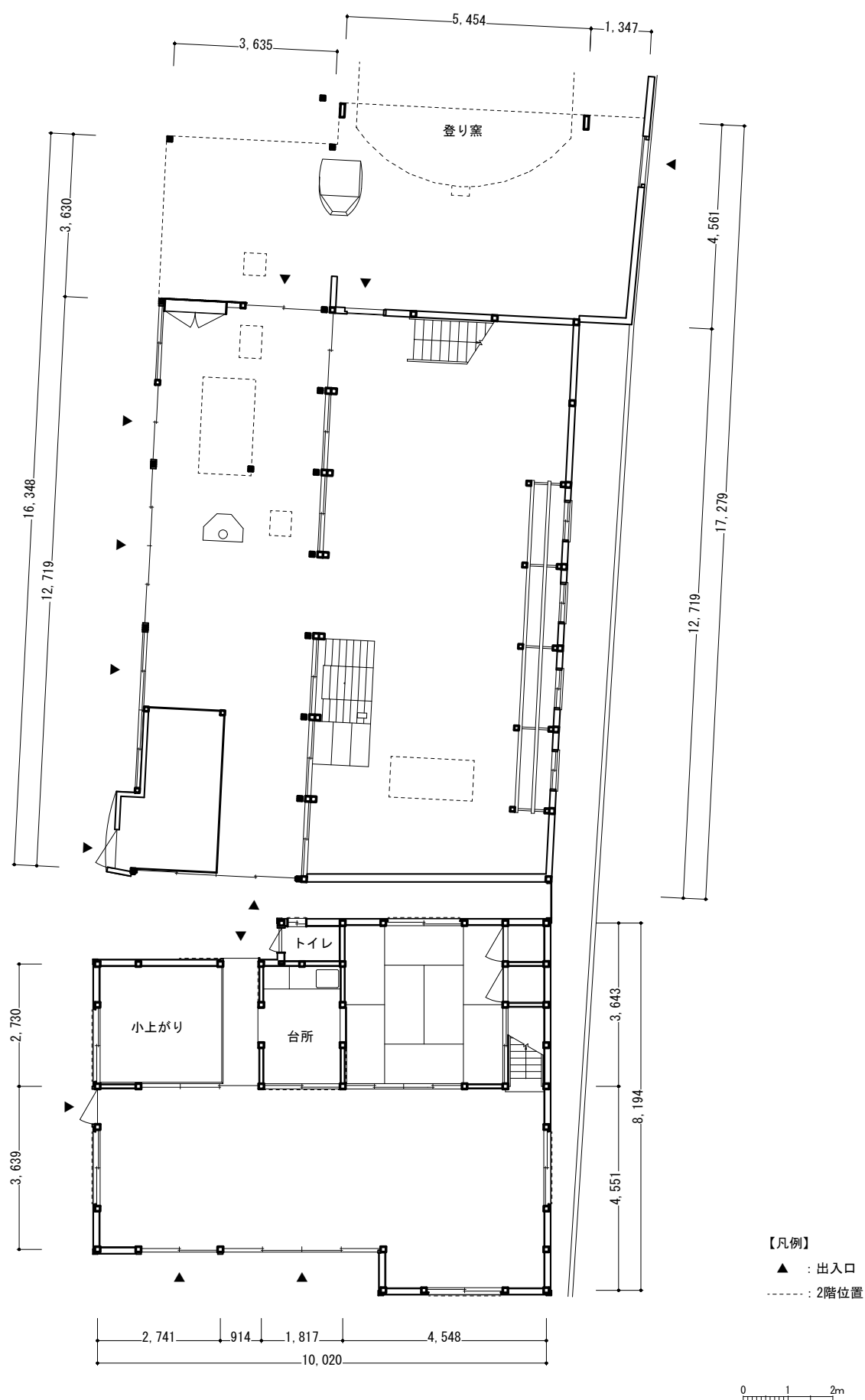
佐藤家 旧店舗・旧工場 1 階平面図
