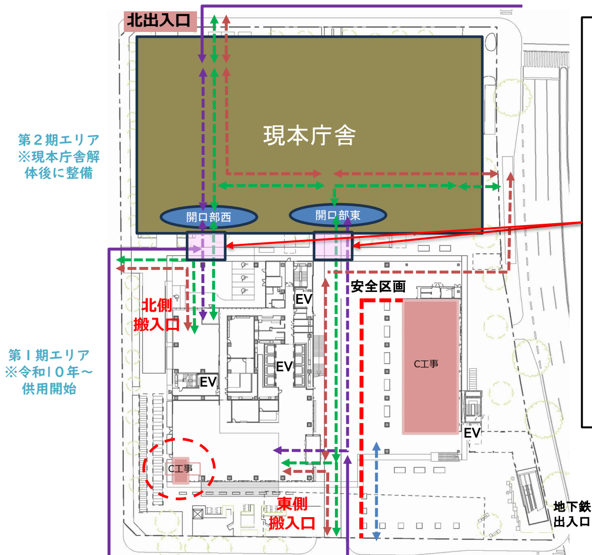
新本庁舎 1階平面図
