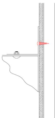
壁：ボードの場合
