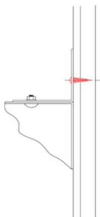
壁：スチールパーティションの場合
