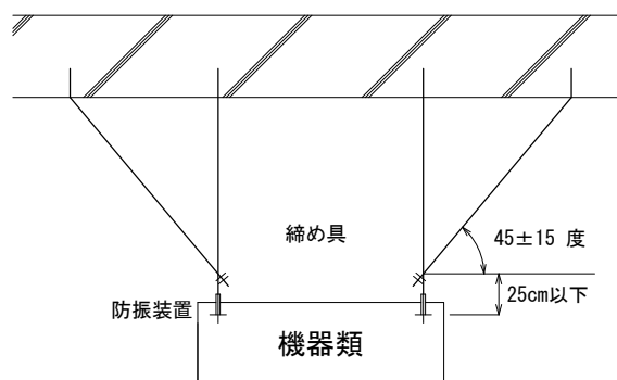
(2) 全ネジボルト放射状の据付け方法
