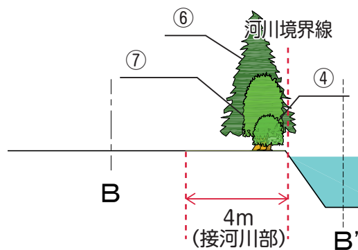
緑化断面図 河川沿い（例）
