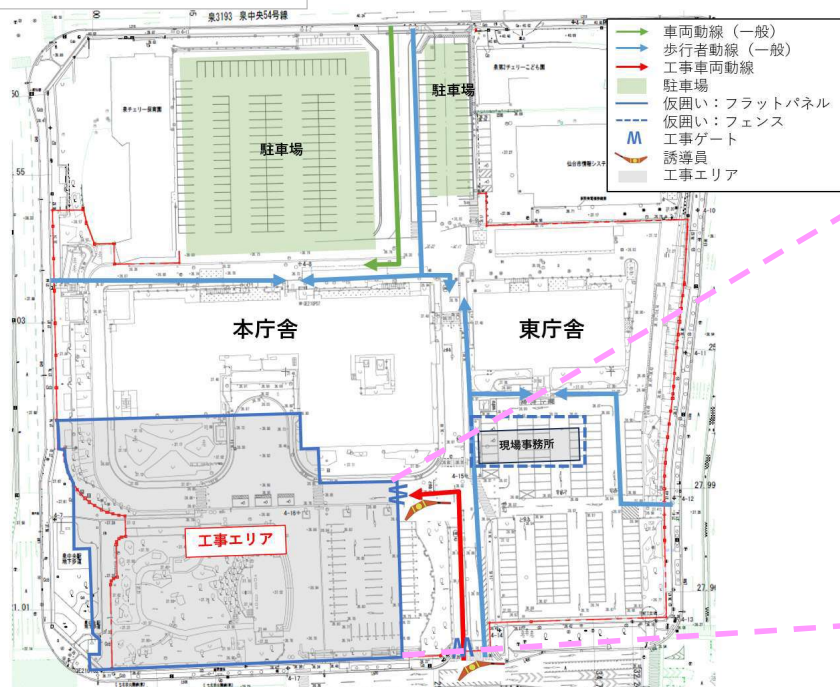
現状配置図(仮設計画)
