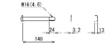
ブラケット取付用ボルト
