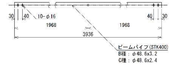
ビームパイプ (STK400)
