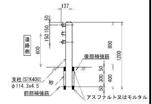
補強筋参考図
