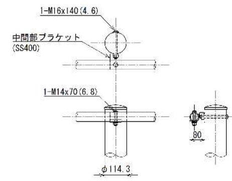
中間部ブラケット (SS400)
