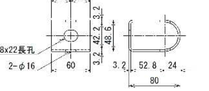
継手ブラケット (SS400)
