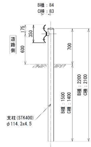
断面図
