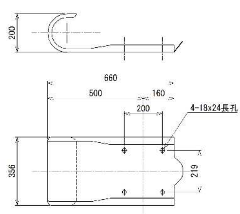
ブラケット (SS400)
