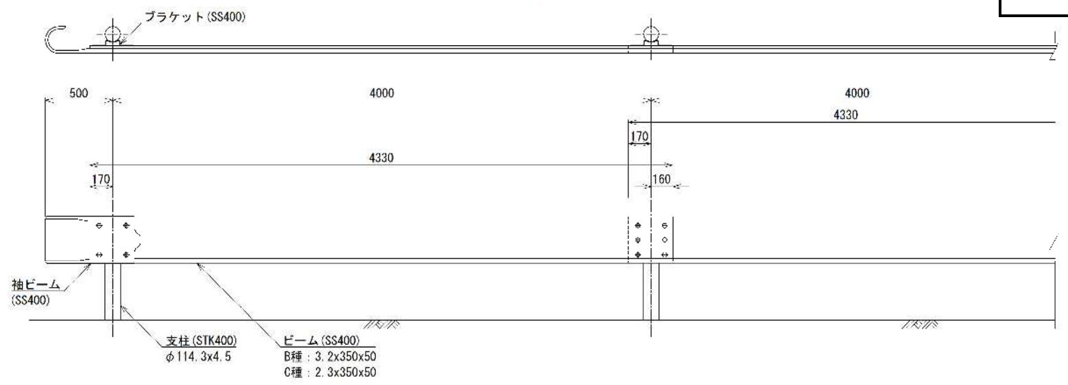
組立図
