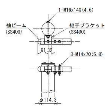
袖ビーム (SS400)
