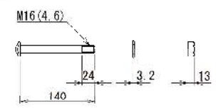
ブラケット取付用ボルト
