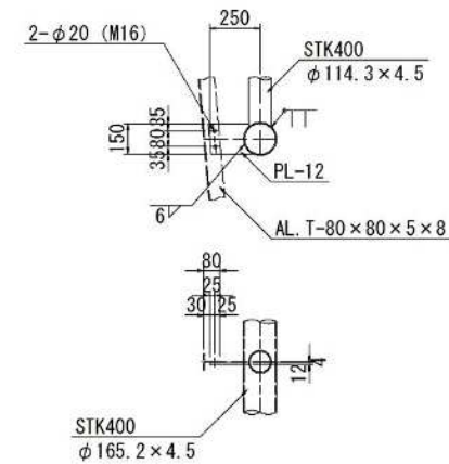
標識板取付部詳細図
