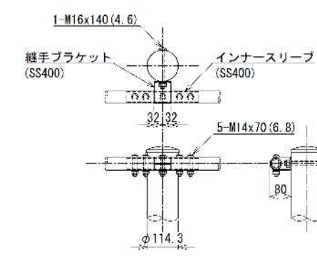
継手ブラケット (SS400)
