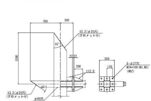
フランジ部詳細図
