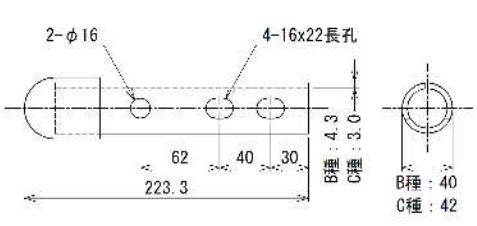
袖ビーム (SS400)
