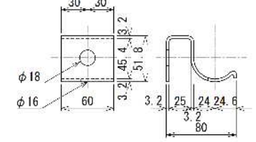
中間部ブラケット (SS400)
