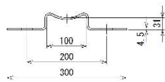
ブラケット(SS400)
