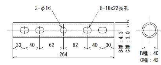
インナースリーブ (SS400)
