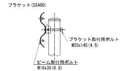
取付詳細図
