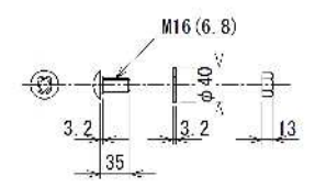
ビーム取付用ボルト
