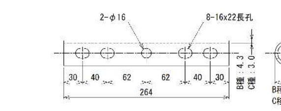
インナー Sleeve (SS400)
