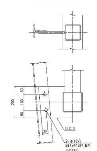
標識板取付部詳細図
