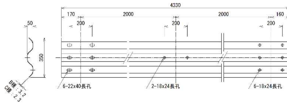
梁(SS400)
