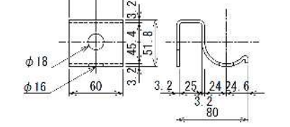
中間部ブラケット (SS400)
