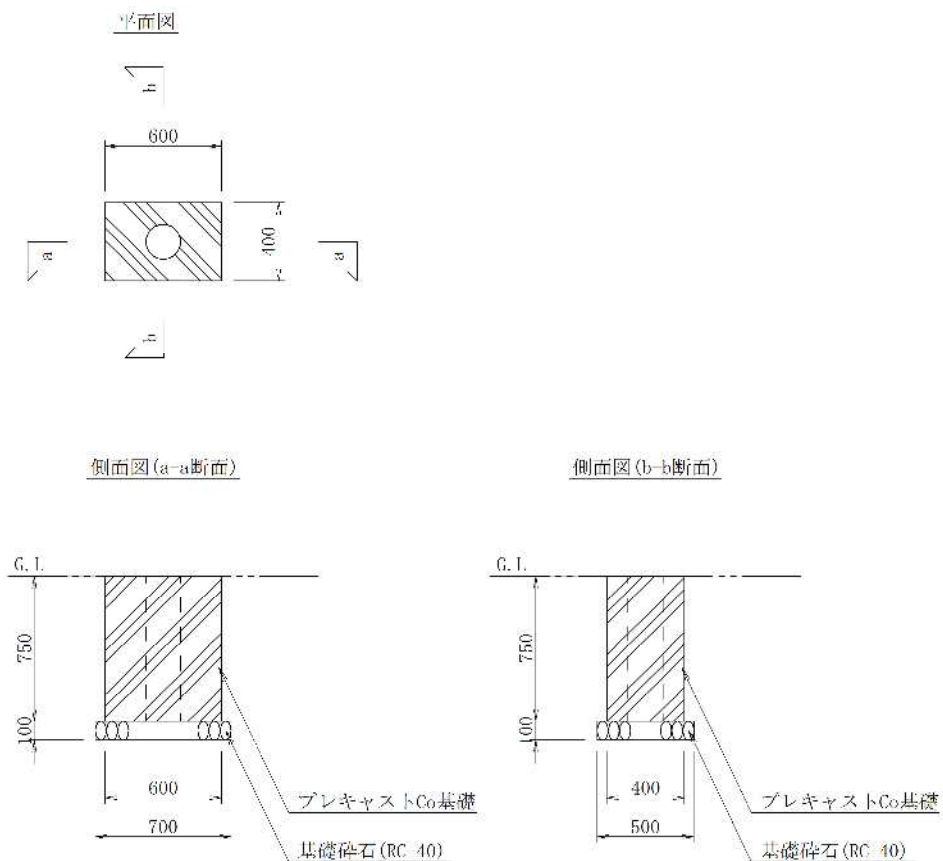
基礎詳細図
