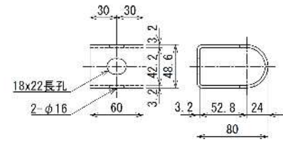
継手ブラケット (SS400)
