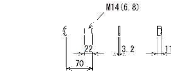
ビーム取付用ボルト
