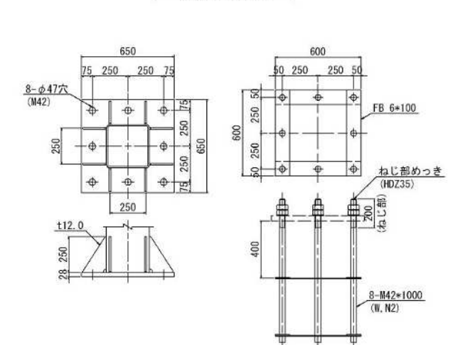
柱脚部詳細図
