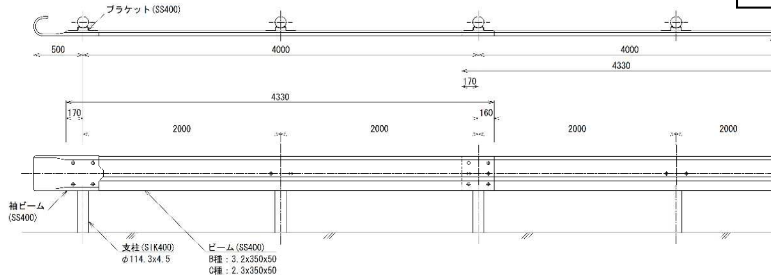
組立図
