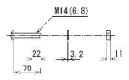
ビーム取付用ボルト
