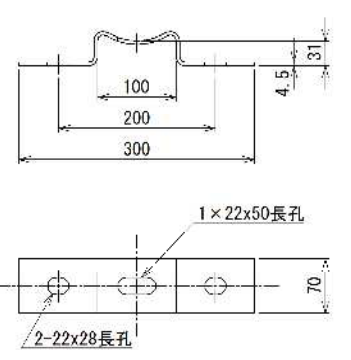
ブラケット (SS400)
