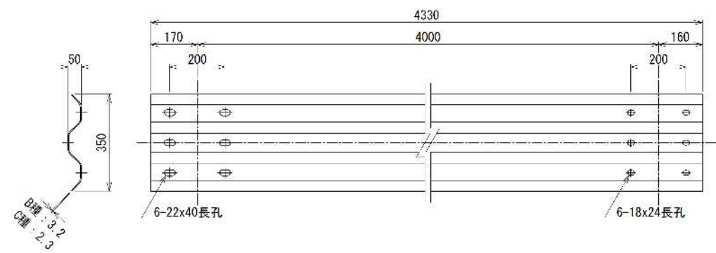
ビーム (SS400)
