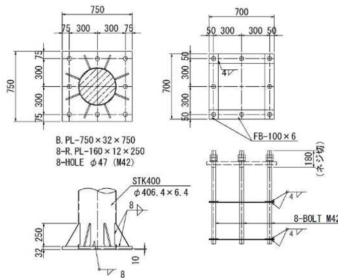
柱脚部詳細図
