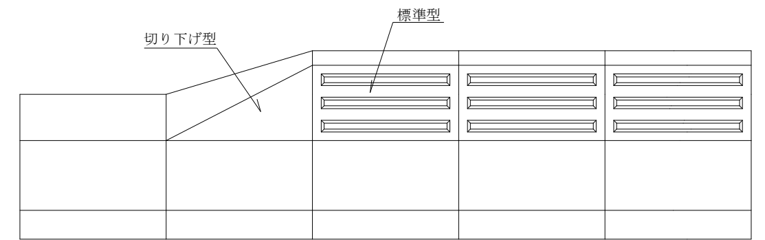
平面図
