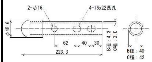
袖ビーム (SS400)
