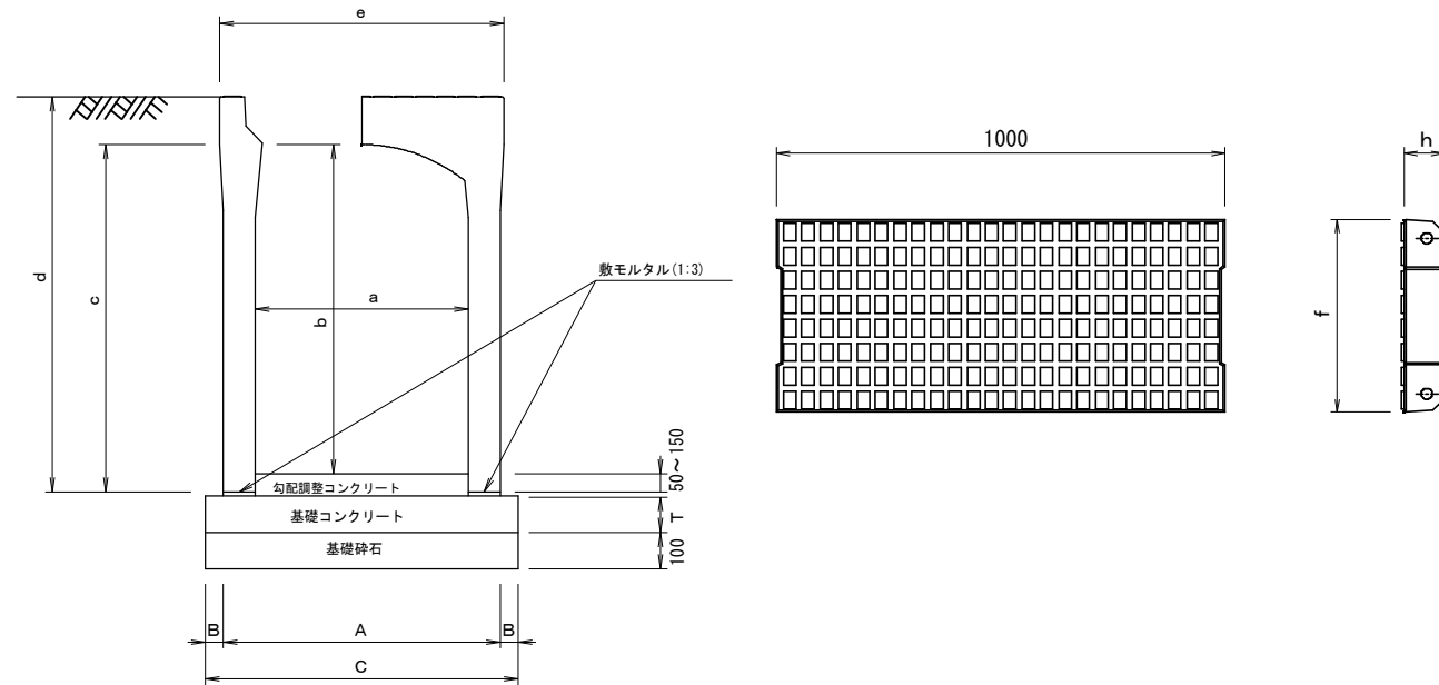
自由勾配側溝用蓋 (L=1000)
