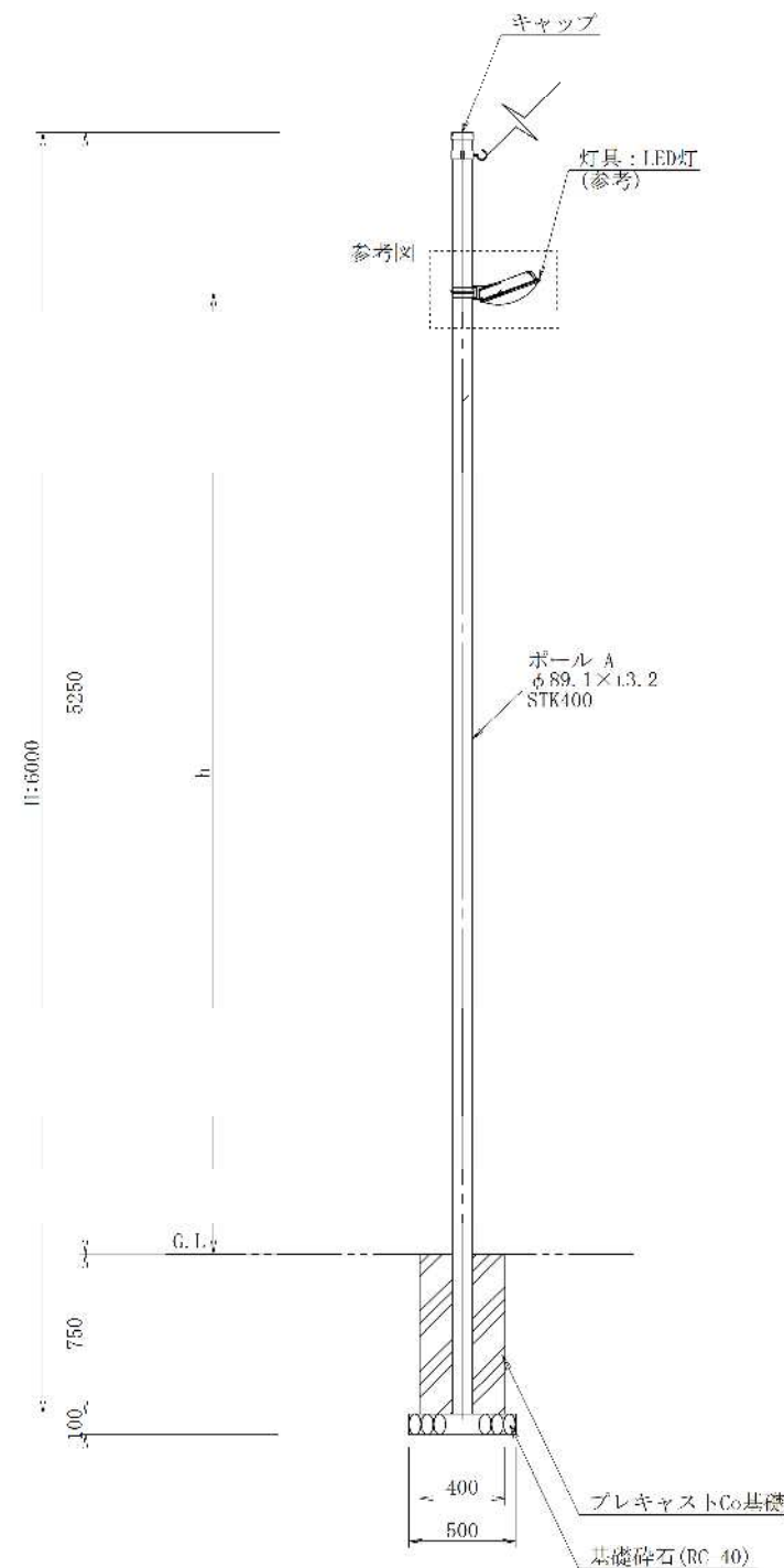
街路灯姿図
