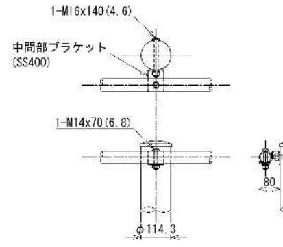
中間部ブラケット (SS400)
