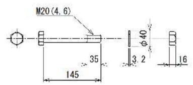
ブラケット取付用ボルト
