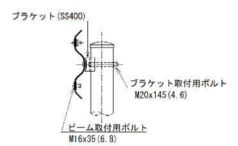
取付詳細図
