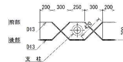
補強筋参考図
