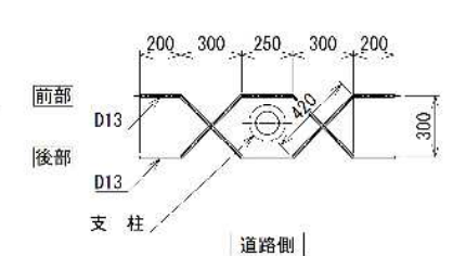
補強筋参考図
