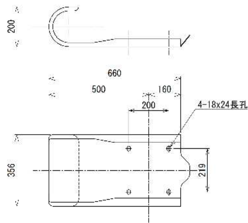
ブラケット(SS400)
