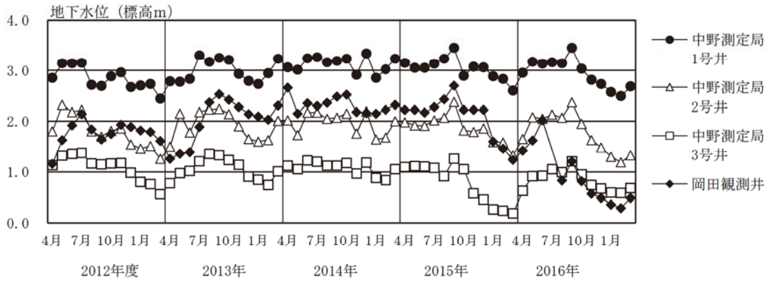
図 6.1.3-7 中野測定局の地下水水位の経年変化
