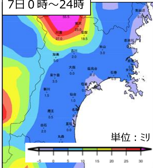
雨量分布図
