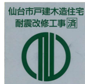
耐震改修済ステッカー
