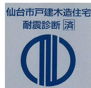
耐震診断済ステッカー
