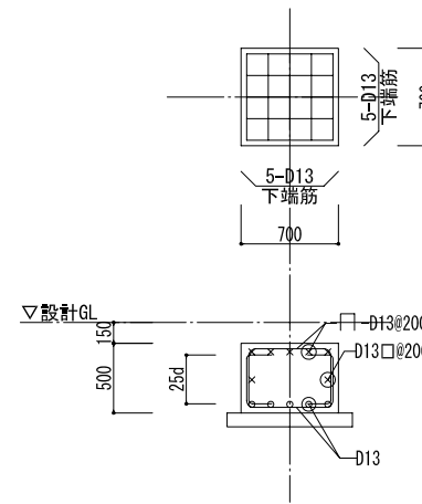
4-1 施設案内サイン基礎
