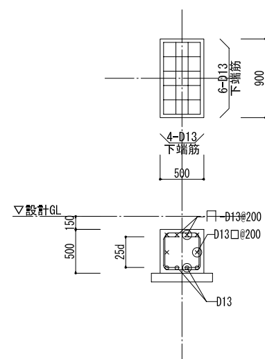
5 連結送水サイン基礎
