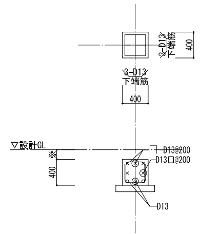
1 施設名サインA基礎
