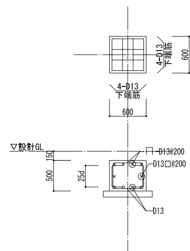
4-2 施設案内サイン基礎
