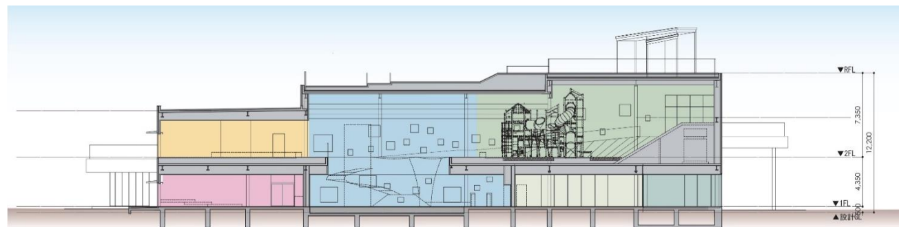
断面図
