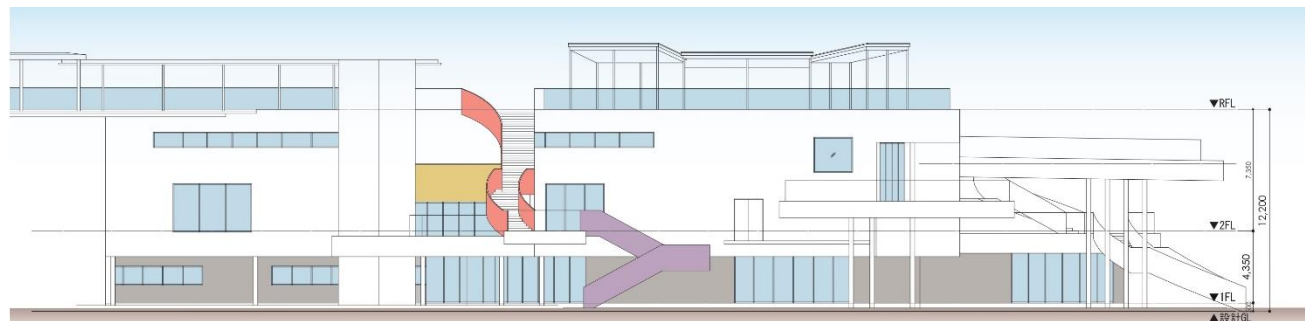
北立面図
