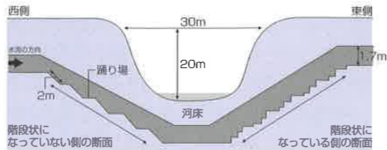
七北田新堰に設けられた伏越の模式図。サイフォンの原理で川底の下に水を通した。
