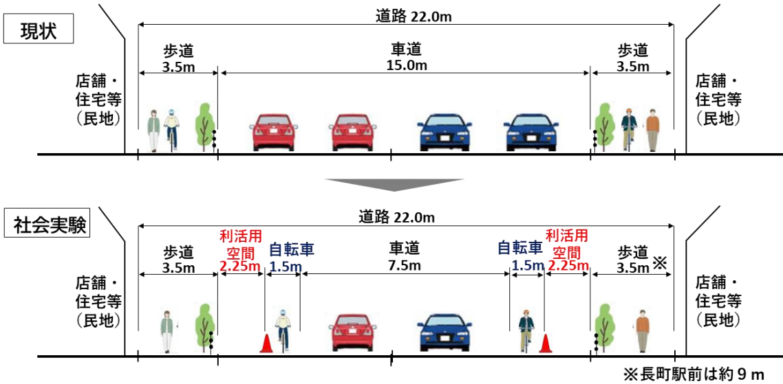
道路断面図
