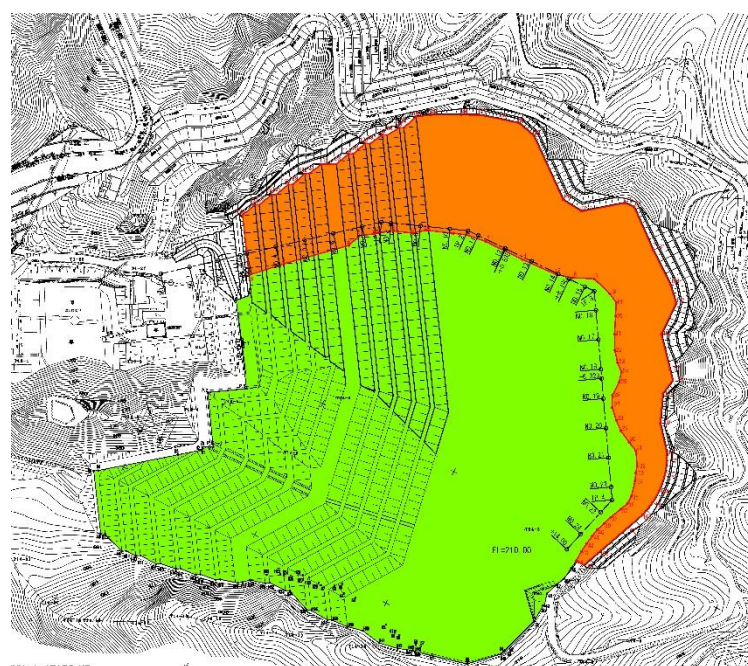
図 変更許可埋立計画図（完了時）
