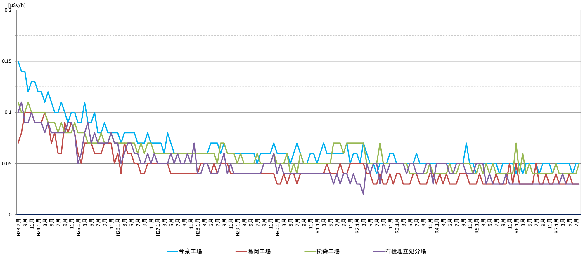
空間放射線量(敷地境界の最大値)の推移 (H23.7~R7.8)
