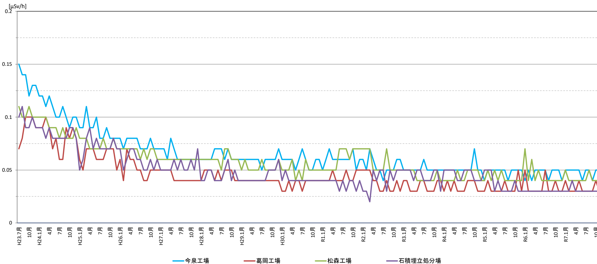
空間放射線量(敷地境界の最大値)の推移 (H23.7~R7.11)
