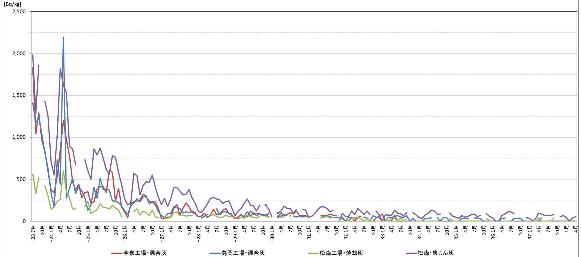
灰の放射性物質濃度の推移 (H23.7~ R8.4)
