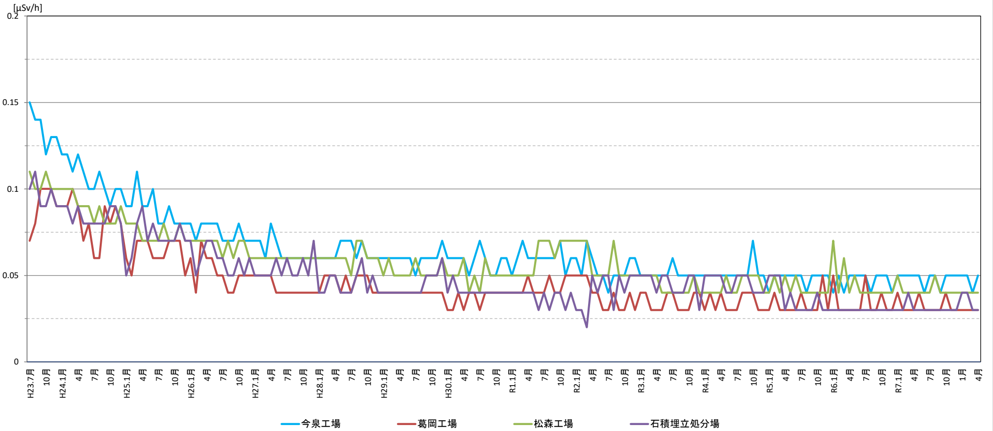
空間放射線量(敷地境界の最大値)の推移 (H23.7~R8.4)
