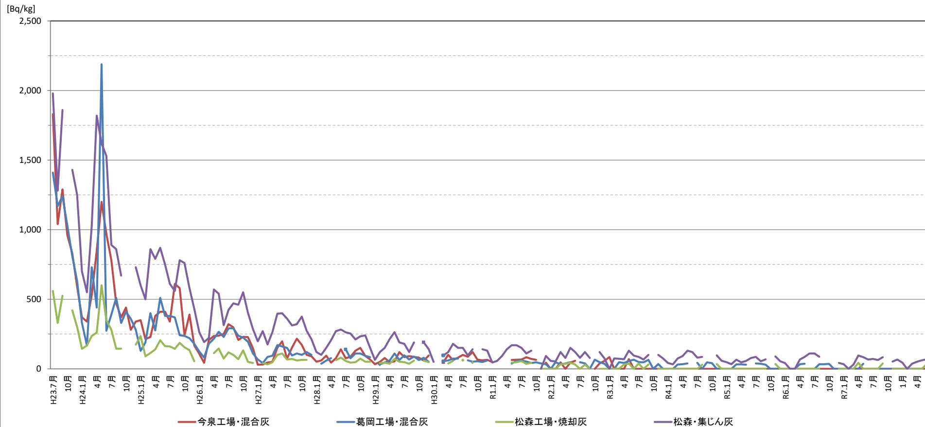
灰の放射性物質濃度の推移（H23.7～ R8.6）
