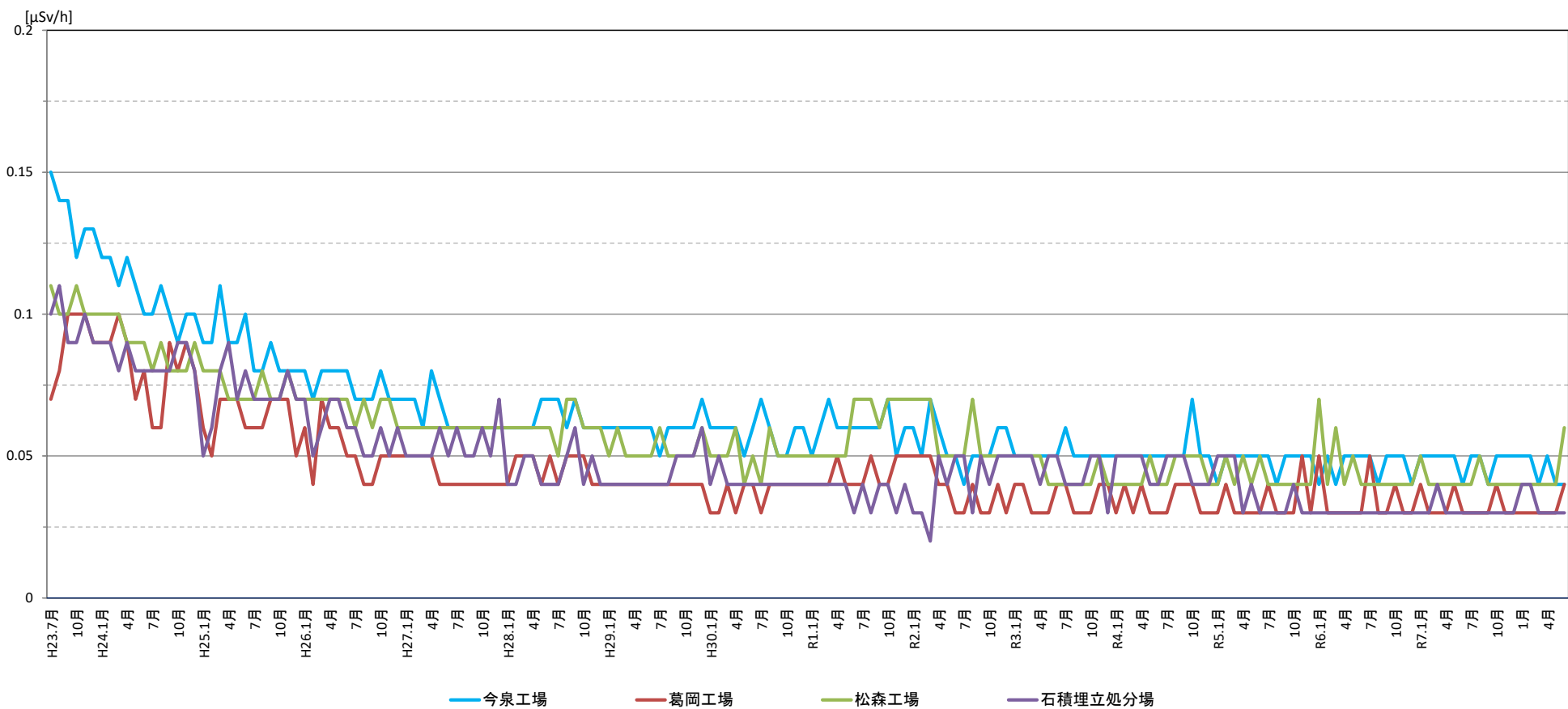
空間放射線量(敷地境界の最大値)の推移 (H23.7～R8.6)
