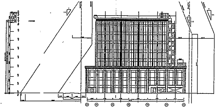
東側立面図
