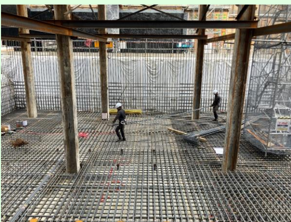
▲鉄筋工事の状況
