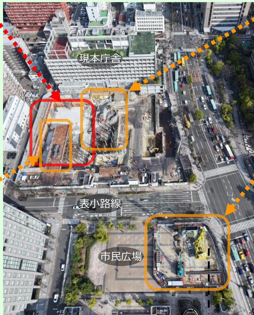
均しコンクリート打設後の様子
