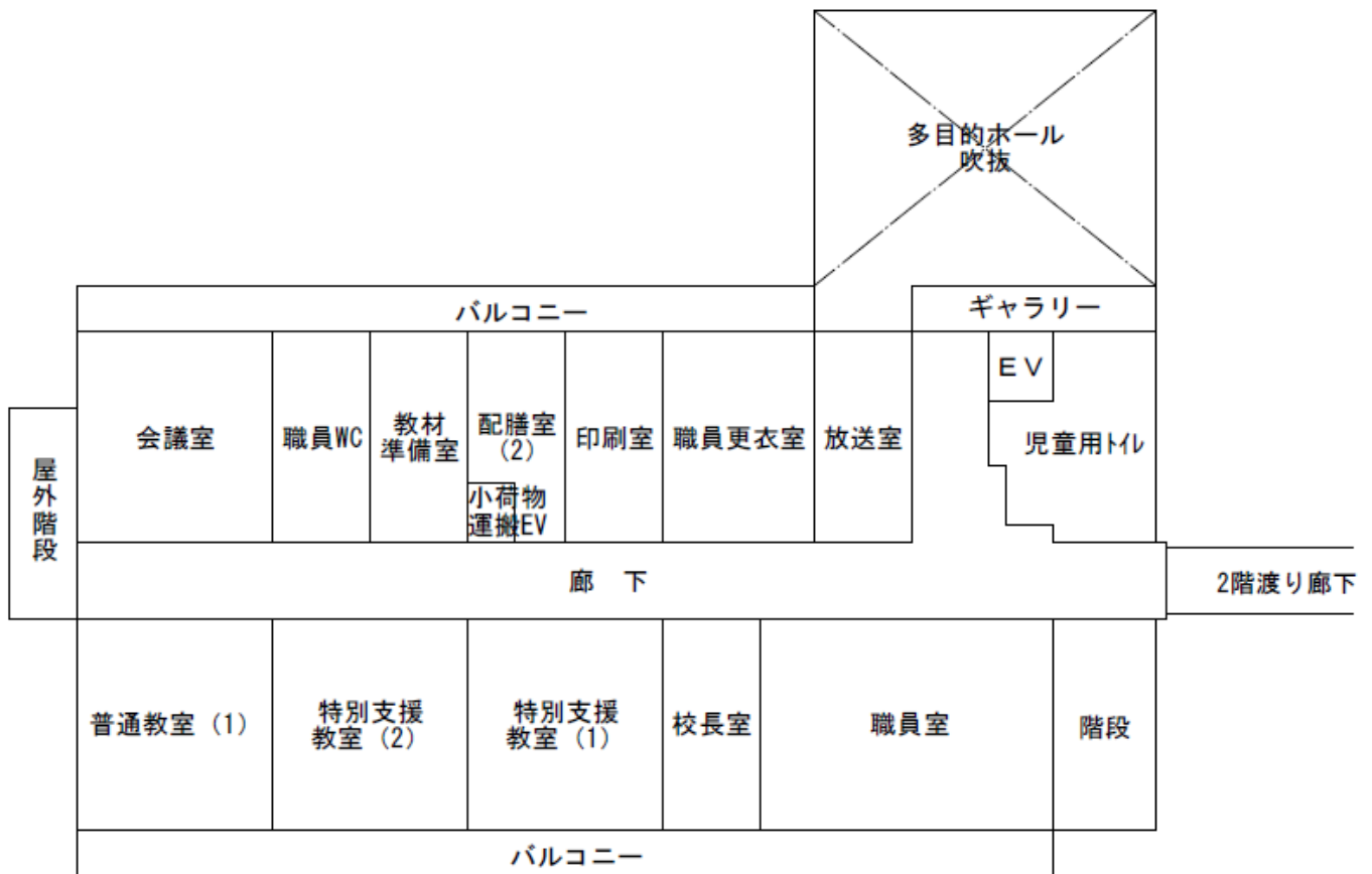
2階平面図
