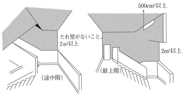
1.2 図1 2 m²開放階段（H14. 11. 28 国告 7）
